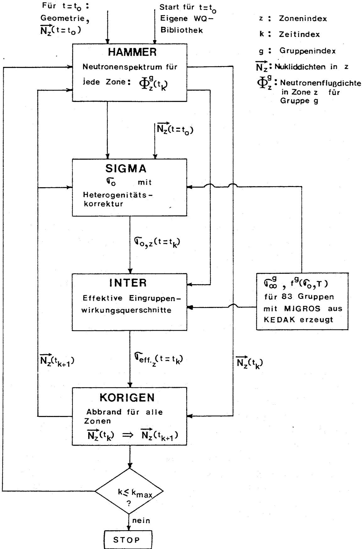
Abb.3.1: Schematische Darstellung des Programms HAMKOR
