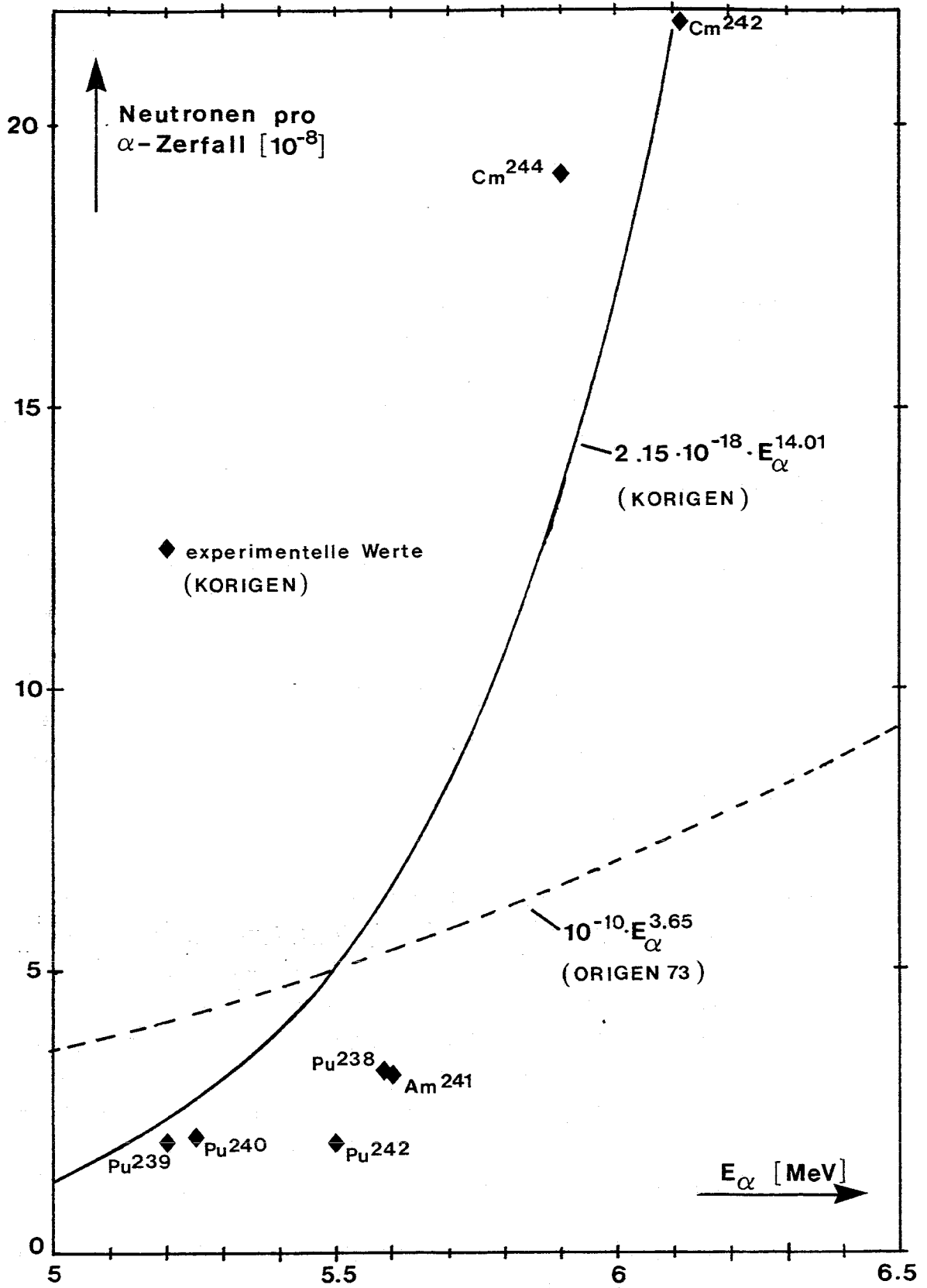
Abb.4.3: Neutronenausbeute aus (\alpha, n) -Reaktionen am Sauerstoff
