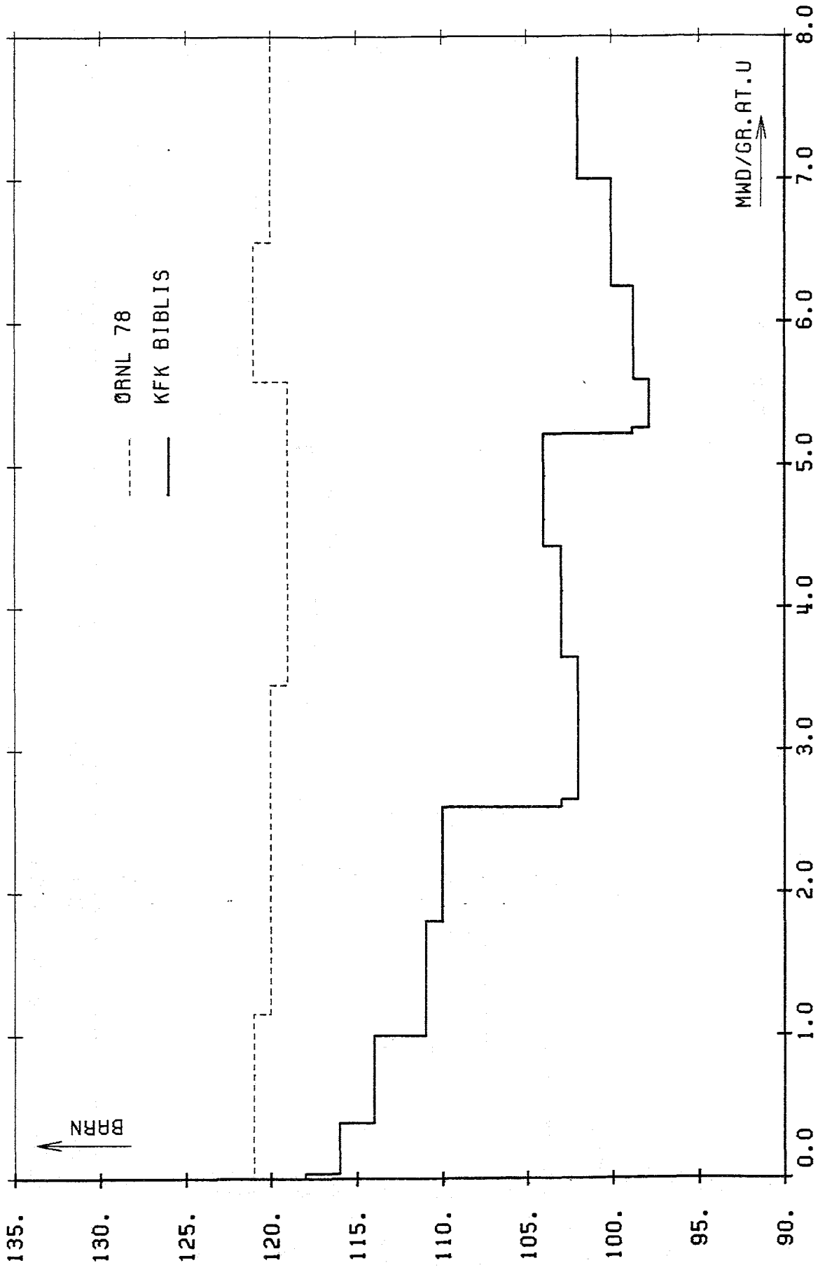
Abb. C. 2--8 PU2h1 SFISS
